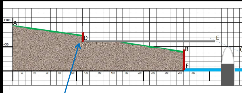
dwarsaanzicht
